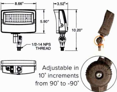
SGF1
